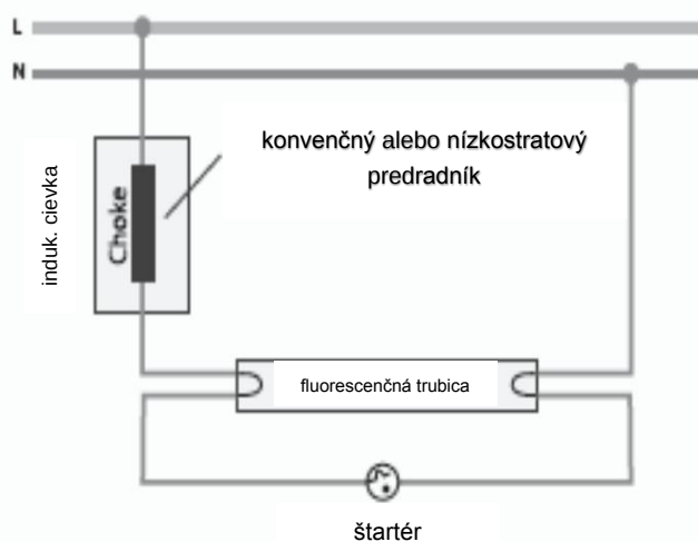
s bežnou fluorescenčnou trubicou
