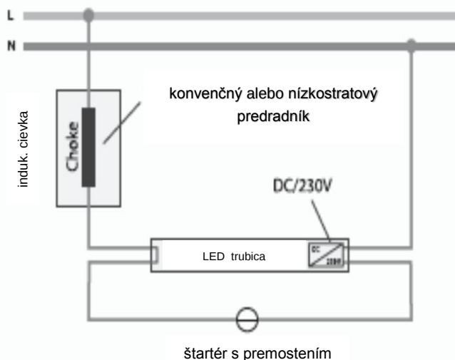
zmena na LED trubicu
